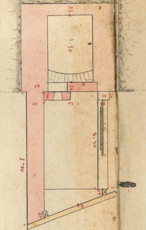
Coupe sur les cabinets et la fosse d'aisance
